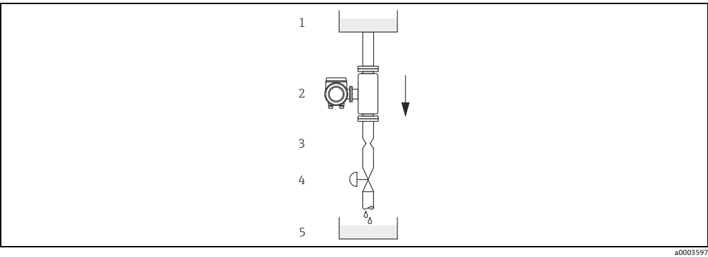
在向下排空管道中安装（例如：批量应用场合）
