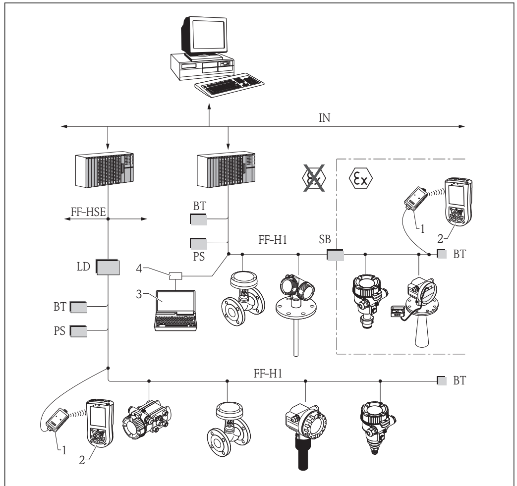
图 26 基金会现场总线(FF)系统架构及其相关部件
