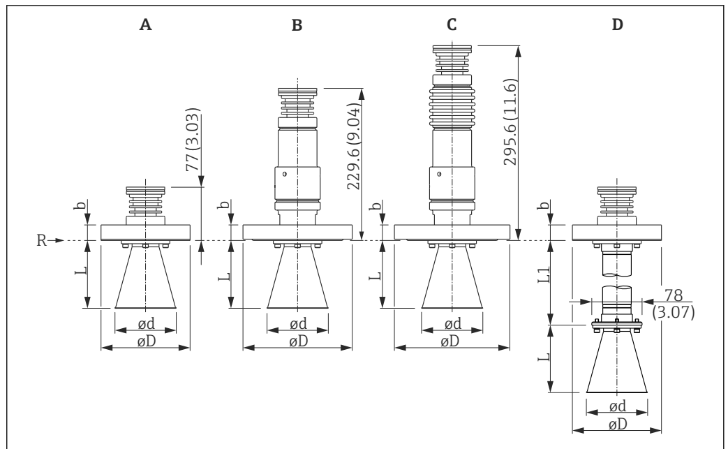
图 23 带螺纹连接的 FMR53 的外形尺寸示意图；单位：mm (in)
