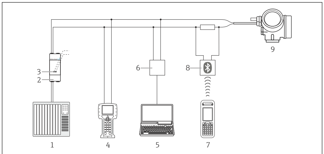
图 25 通过 HART 通信进行远程操作
