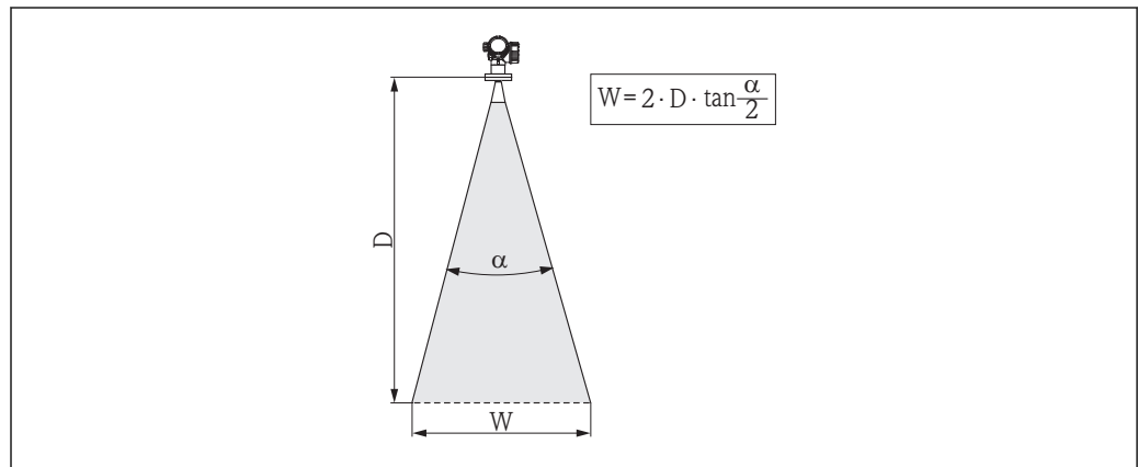
图 10 波束角 \alpha 、距离 D 和波束宽度 W 的关系示意图
