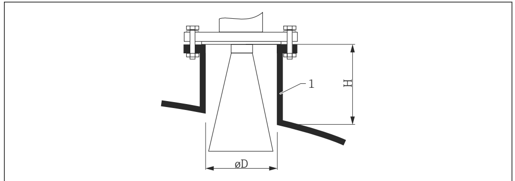
图 12 喇叭天线的安装短管长度和管径(FMR54)示意图
