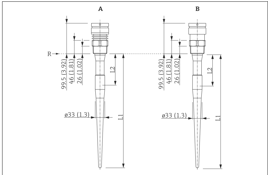
图 22 带螺纹连接的 FMR53 的外形尺寸示意图；单位：mm (in)
