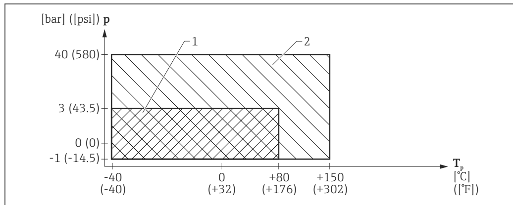
图 15 FMR53: 允许过程温度和过程压力范围
